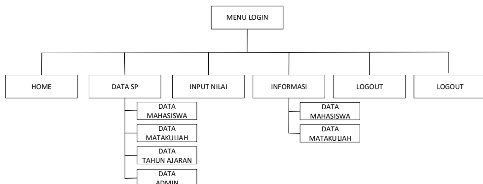
Gambar 3.6 Struktur Menu Admin
