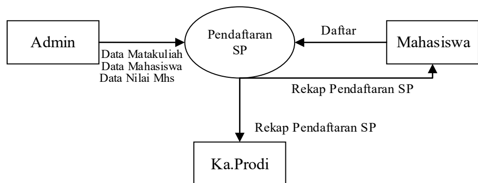
Gambar 3.2 Diagram Konteks
